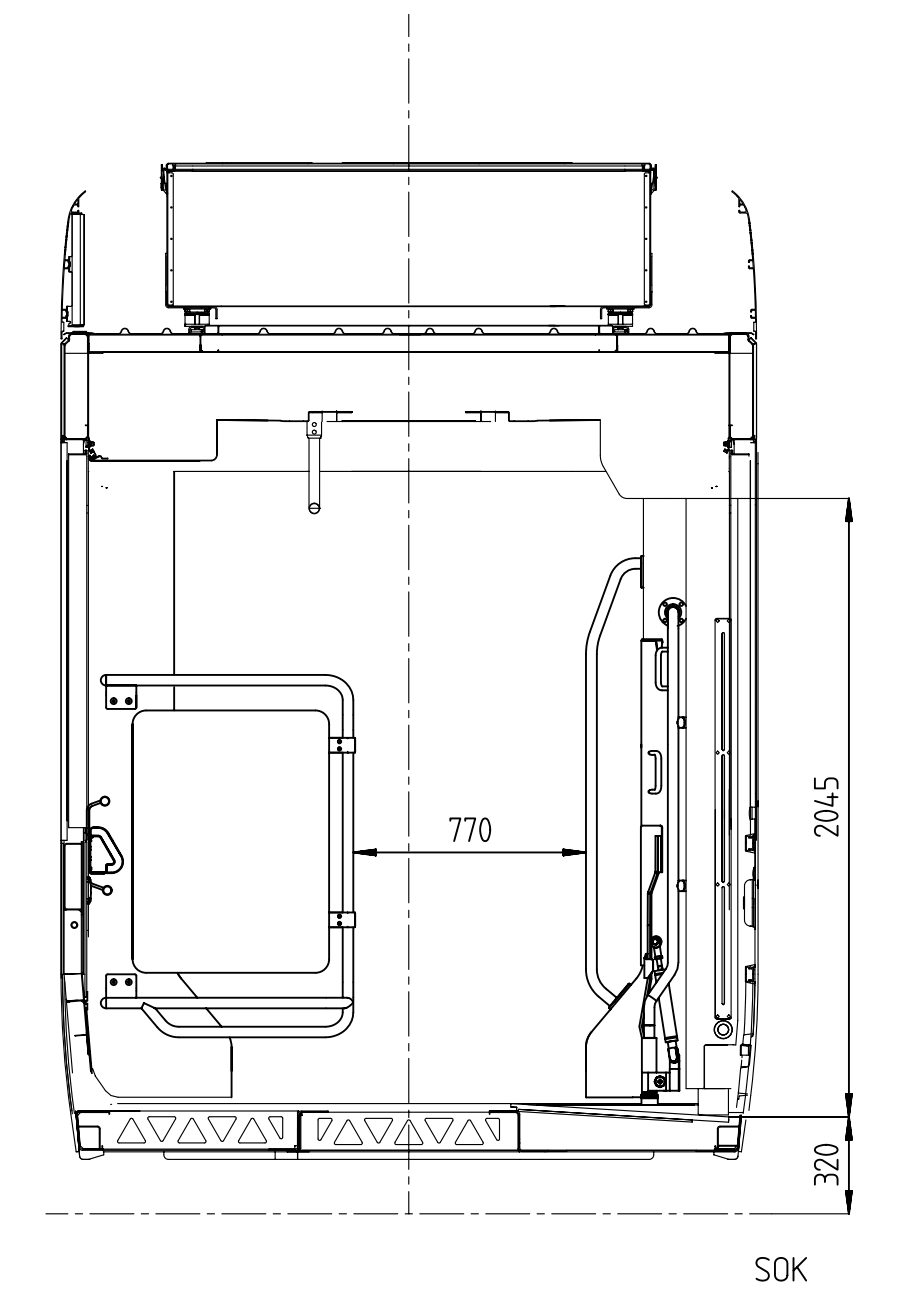
SCHNITT C
