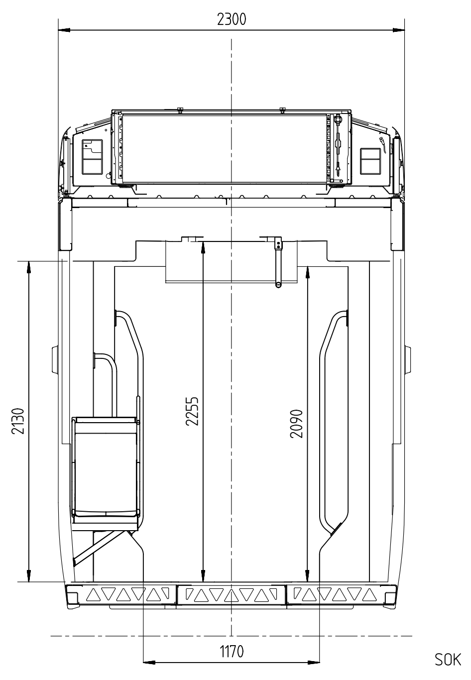
SCHNITT A
