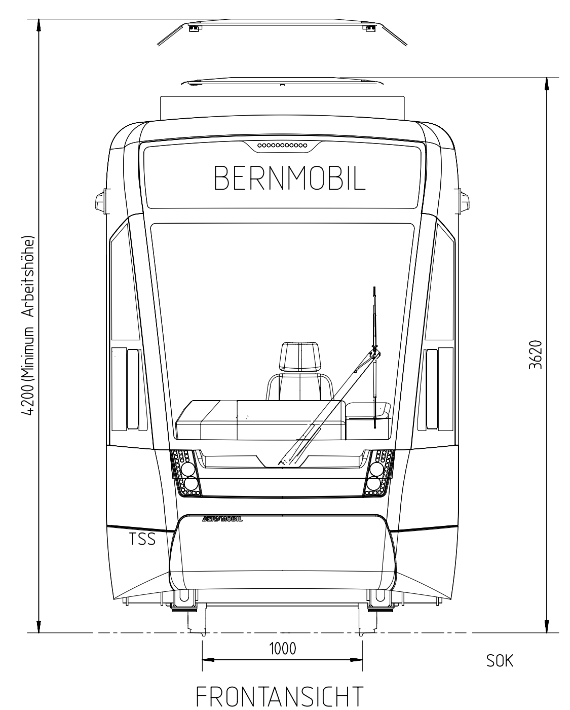
FRONTANSICHT
