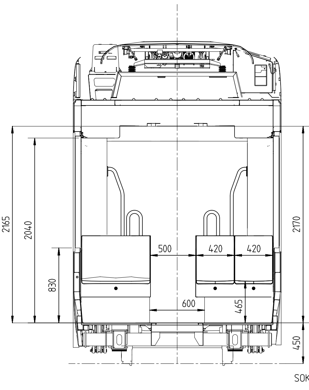
SCHNITT B
